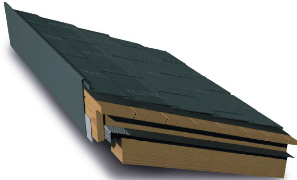
PULTDACHABSCHLUSS HINTERLÜFTET
