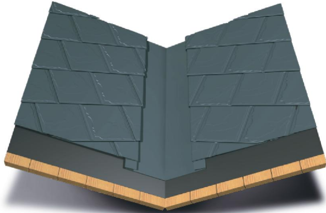
3D SCHNITT VERTIEFTE KEHLE VARIANTE 2
