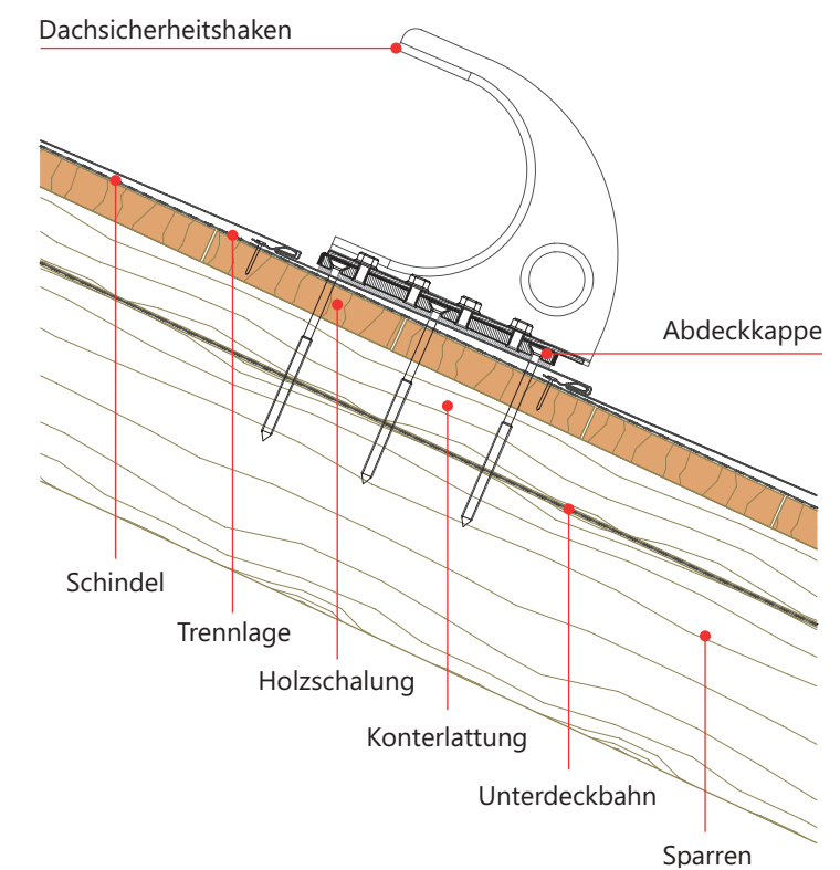
DETAIL DACHSICHERHEITSHAKEN
