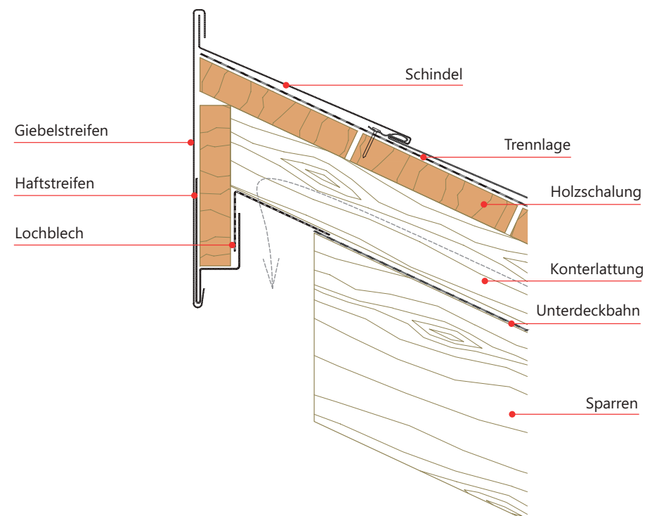
DETAIL PULTDACHABSCHLUSS HINTERLÜFTET
