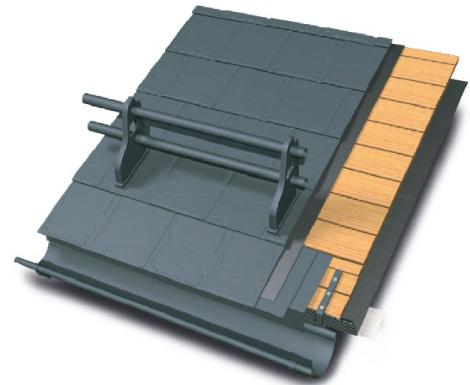
DETAIL SCHNEEFANG
