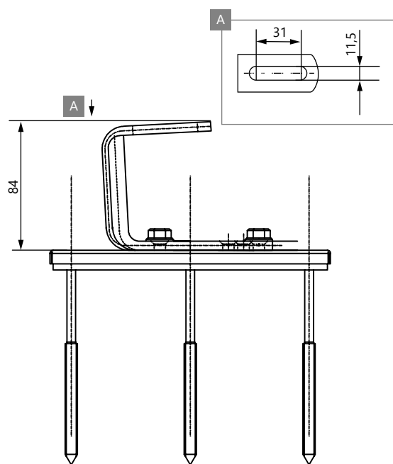
Maße sind ca. - Angaben in mm
